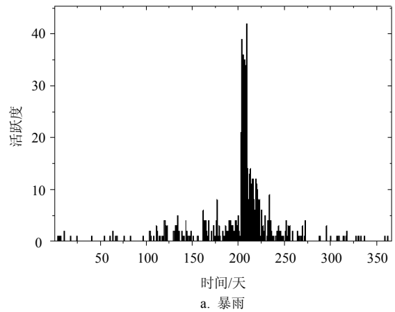
a. 暴雨
